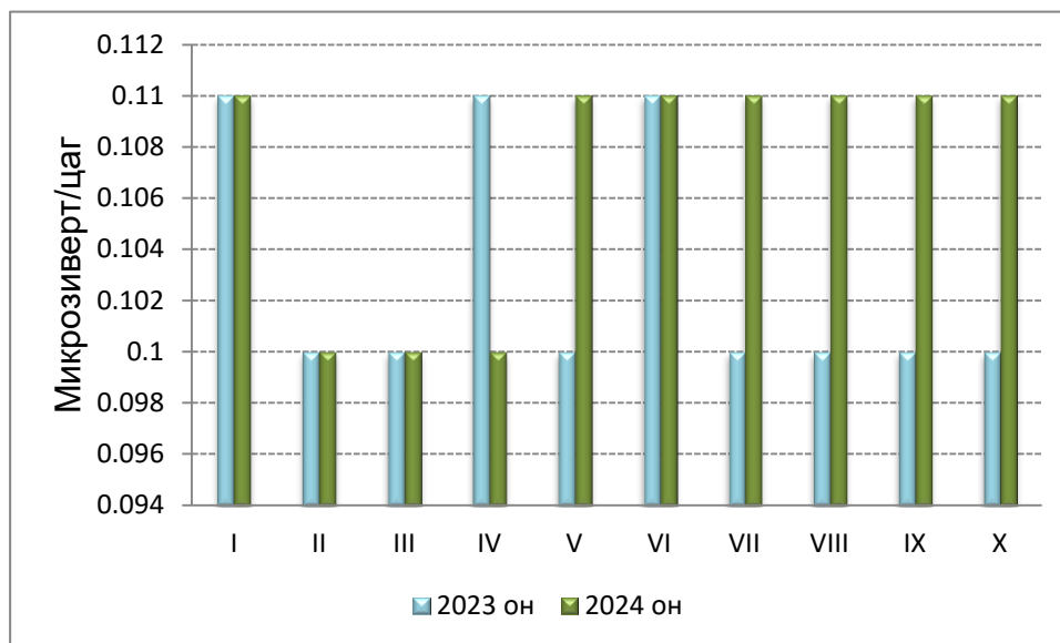
График3. Улиастай сумын 2023, 2024 оны цацрагийн хэмжилтийн утга
